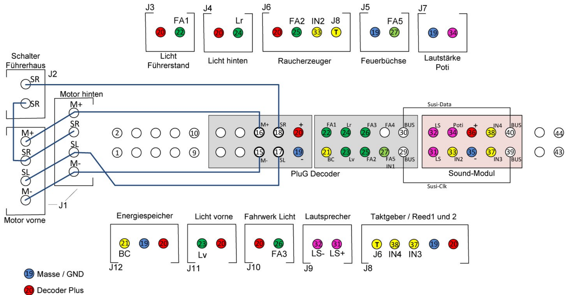
Train Line Gartenbahnen HSB-Mallet PluG-S20 Schnittstelle
