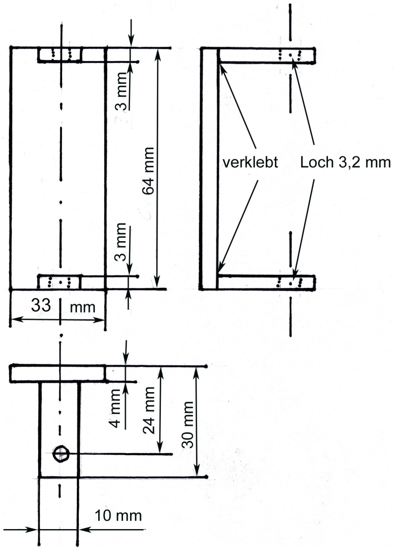
Maßskizze Achshalter Mittelachse (Abmaße für Nenngroße 11m)
